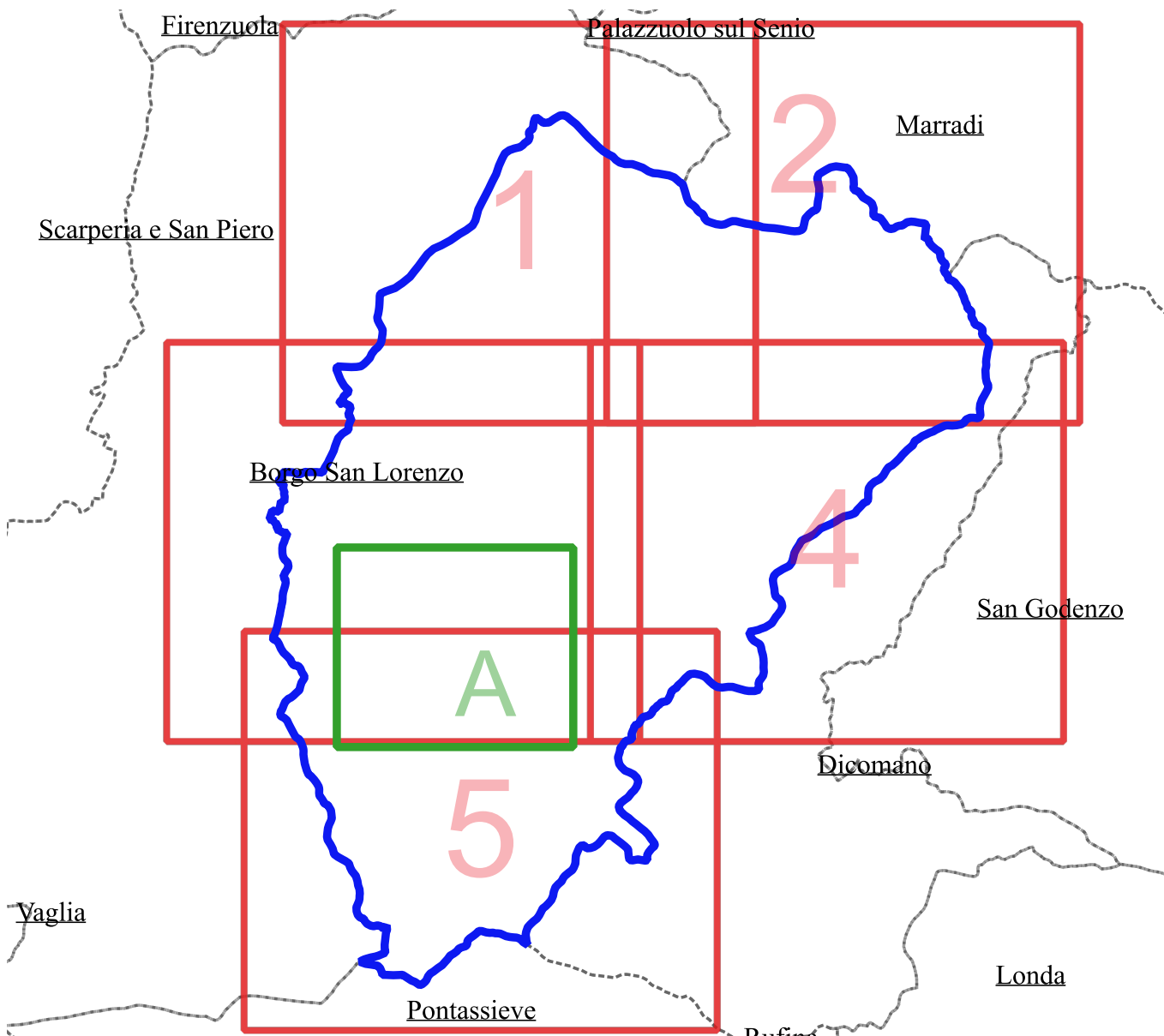
TAV. 12: Pericolosità sismica - Passo 002 e Studi MS Quadrante 2
